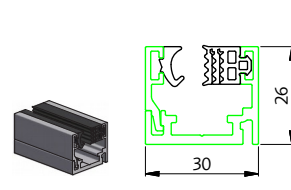
PROFIL D'ENCADREMENT
